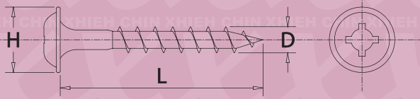
B1038 D*L*H
