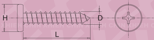
B1020 D*L*H
