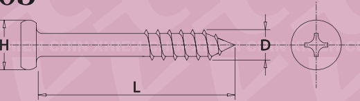
B1003 D*L*H
