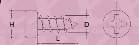
B1030 D*L*H
