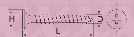
B0361 D*L*H
