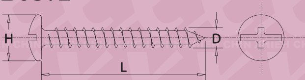
B0372 D*L*H
