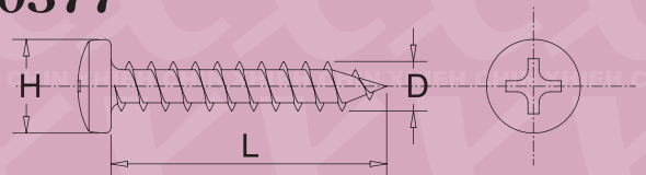
B0377 D*L*H
