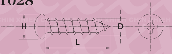
B1028 D*L*H
