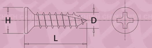
B1019 D*L*H
