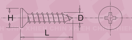
B0369 D*L*H
