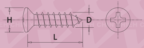
B0376 D*L*H
