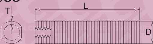
A1055 D*L*T
