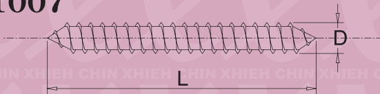
B1007 D*L
