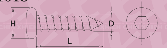
B1015 D*L*H
