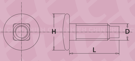
B1035 D*L*H
