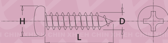
B1022 D*L*H
