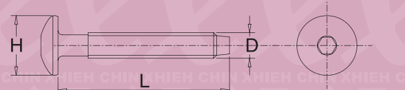
B1046 D*L*H
