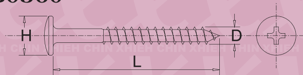
B0360 D*L*H
