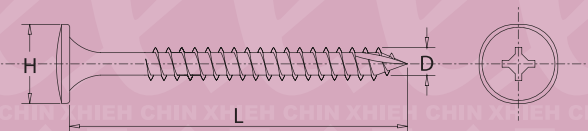
B1042 D*L*H
