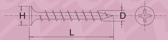
B0359 D*L*H
