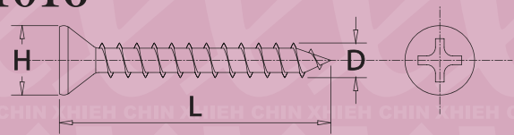
B1016 D*L*H
