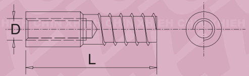
B0358 D*L
