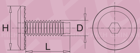
B1050 D*L*H
