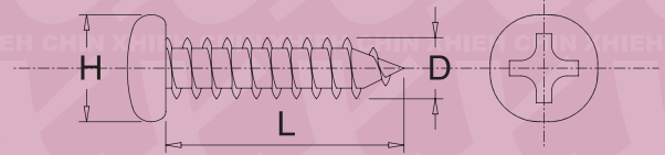
B1023 D*L*H
